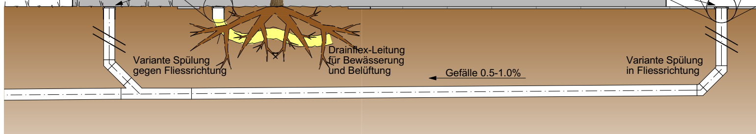
Schnitt
